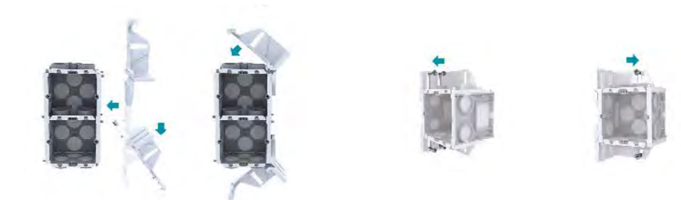
Fixation de plusieurs boîtes Bevestiging van meerdere inbouwdozen
